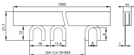
Рисунок 4 – Шина типа FORK 2P 63 А шаг 18 мм
