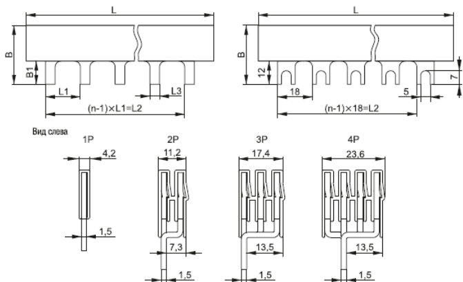
Рисунок 9 – Шина типов PIN и FORK 100 А
