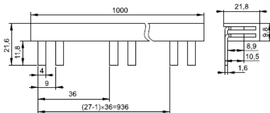
Рисунок 12 – Шина соединительная PIN 63A 54 мод. для диф. авт. (1 м)
