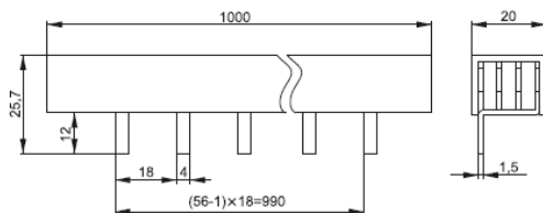
Рисунок 7 – Шина типа PIN 4P 63 А шаг 18 мм
