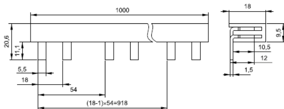
Рисунок 11 – Шина соединительная PIN 63A 36 мод. для АД12 (1 м)
