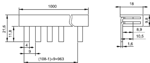
Рисунок 10 – Шина соединительная PIN 63A 108 мод. для АВДТ32М (1 м)
