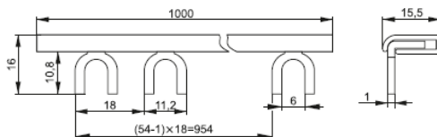
Рисунок 2 – Шина типа FORK 1P 63 А шаг 18 мм
