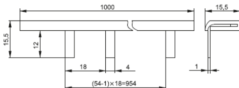
Рисунок 1 – Шина типа PIN 1P 63 А шаг 18 мм s/n AN0804.00001247
