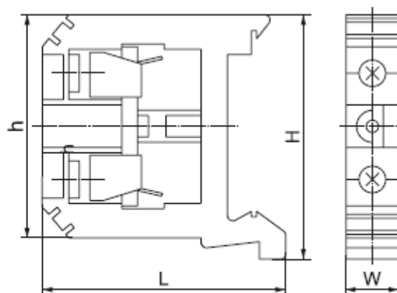
Рисунок 2 – ЗНИ для фазных проводников
