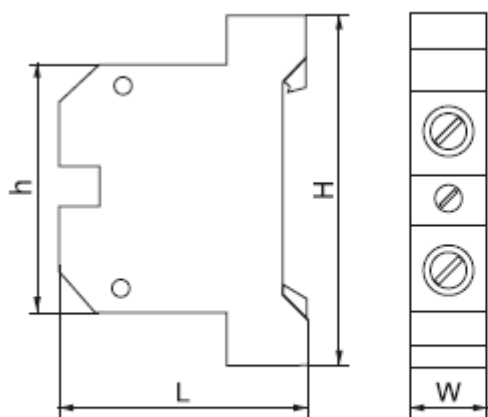
Рисунок 1 – ЗНИ для РЕ и PEN проводников
